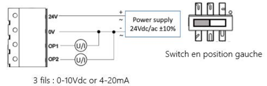
Schéma de raccordement :
