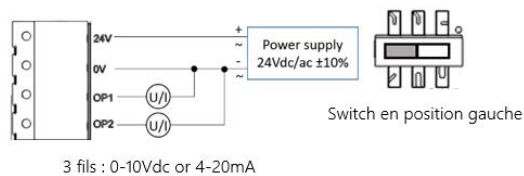
Schéma de raccordement :
