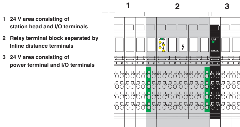
Dessin schématique
